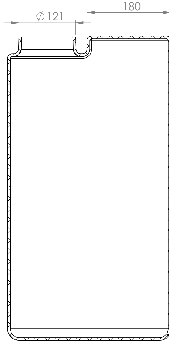
KESİT A-A ÖLÇEK 1 : 5
