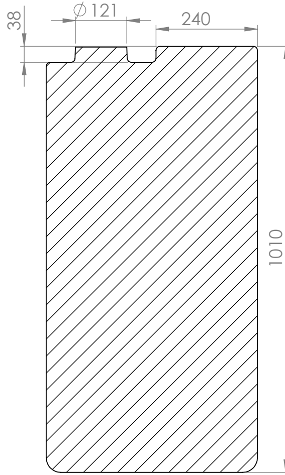
KESİT A-A ÖLÇEK 1 : 9
